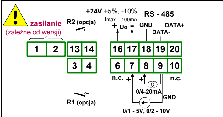
Rys. 4.5. Opis wyprowadzeń dla wersji z wyjściami przekąźnikowymi
