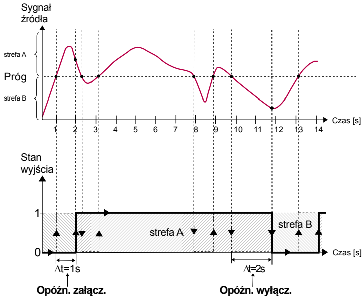
Rys. 7.97. Zasada pracy przełączników wirtualnych dla przykładowych ustawień czasowych: Opóźn.załącz.= 1 sec., Opóźn.wyłąc.= 2 sec.
