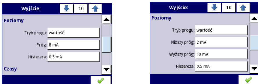
Rys. 7.96. Ustawienia poziomów dla trybu nad progiem i pod progiem (lewy rys.) oraz wewnątrz zakresu i poza zakresem (prawy rys.)
