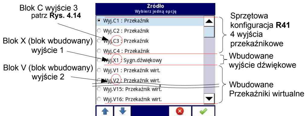
Rys. 7.61. Przykładowe opcje dla Źródła w trybie Podgląd wyjścia
