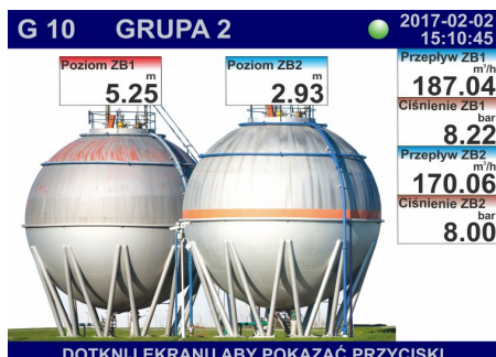
Rys. 7.150. Przykładowe wizualizacje trybu SCADALite
