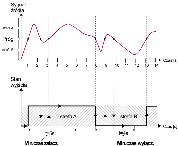
Rys. 7.101. Zasada pracy wyjść przekaźnikowych dla przykładowych ustawień czasowych: Min.czas załącz. = 5 sec., Min.czas wyłącz. = 4 sec.
