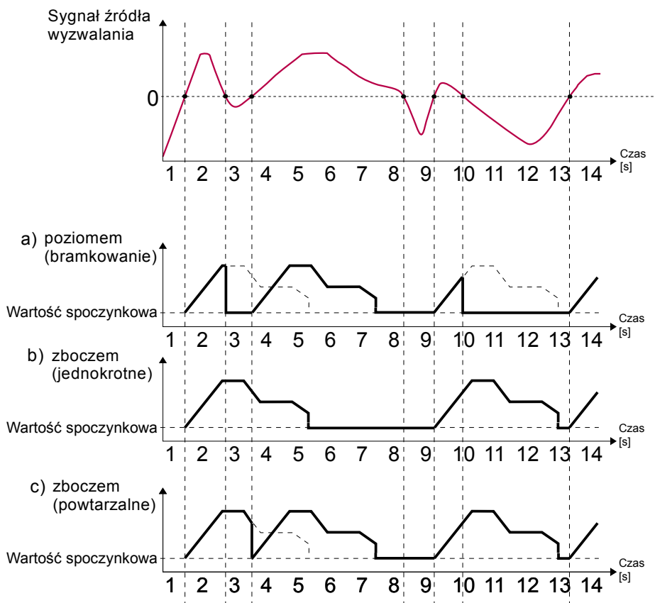
Rys.7.120. Przykładowe przebiegi wyjściowe Profilu zdefiniowanego na Rys.7.119 wyzwalanego sygnałem źródła wyzwalania dla Trybu wyzwalania: poziomem (bramkowanie) , zбочem (jednokrotne) , zбочem (powtarzalne)
