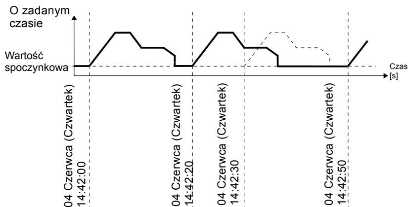
Rys.7.122. Przebieg sygnału wyjściowego dla trybu o zadanym czasie i parametrów czasowych zgodnych z Rys.7.121
