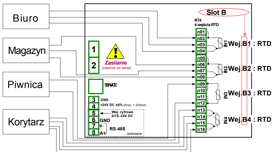
Rys. 7.81. Schemat połączeniowy dla modułu RT4
