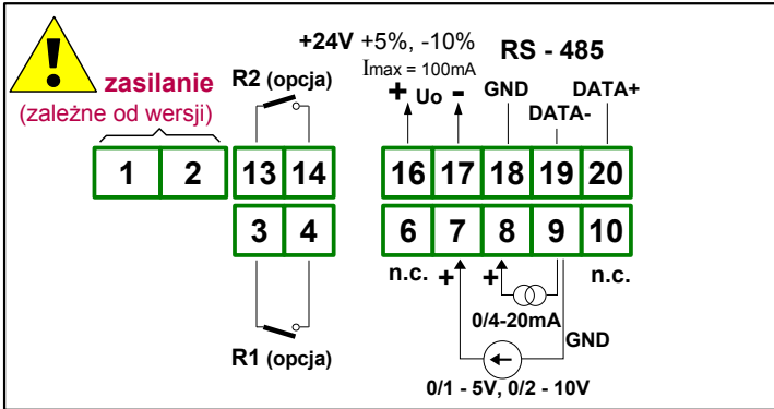
Rys. 4.5. Opis wyprowadzeń dla wersji z wyjściami przełącznikowymi
